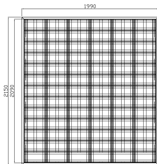
VISTA FRONTAL FURAÇÃO DOS MÓDULOS
