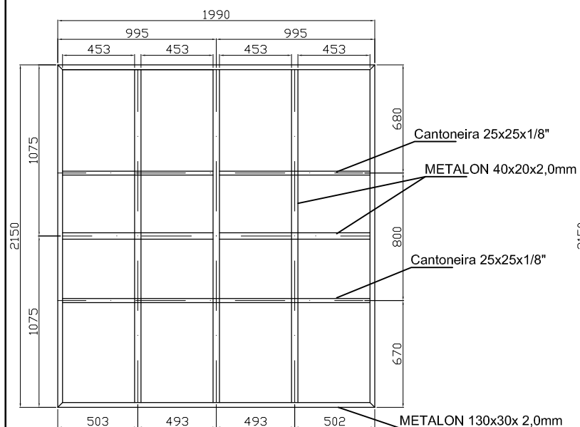
VISTA FUNDO
