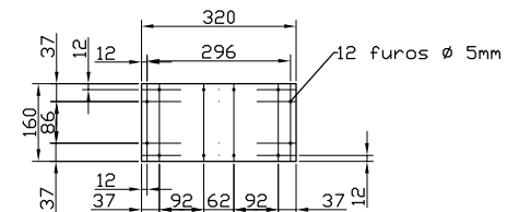
GABARITO DE FURAÇÃO
