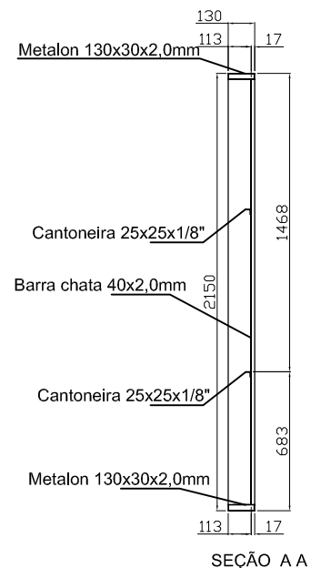
SEÇÃO A A
